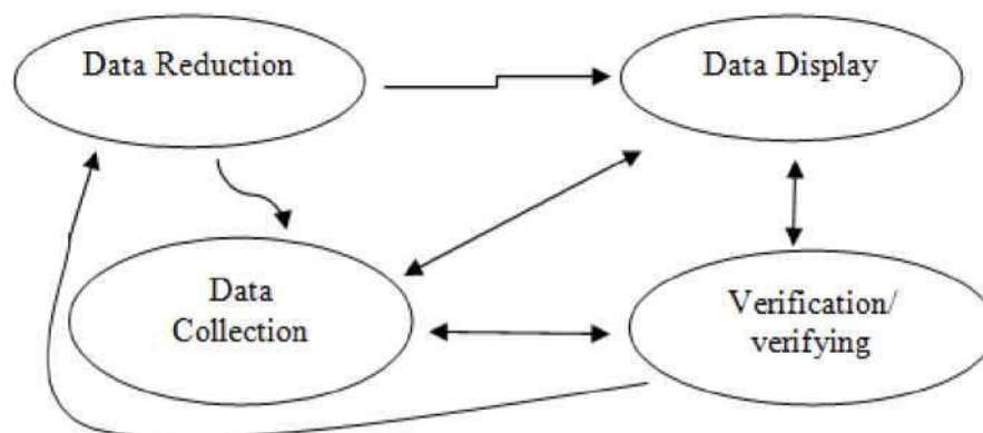
Gambar 3.1 Model Analisis Data Interaktif
