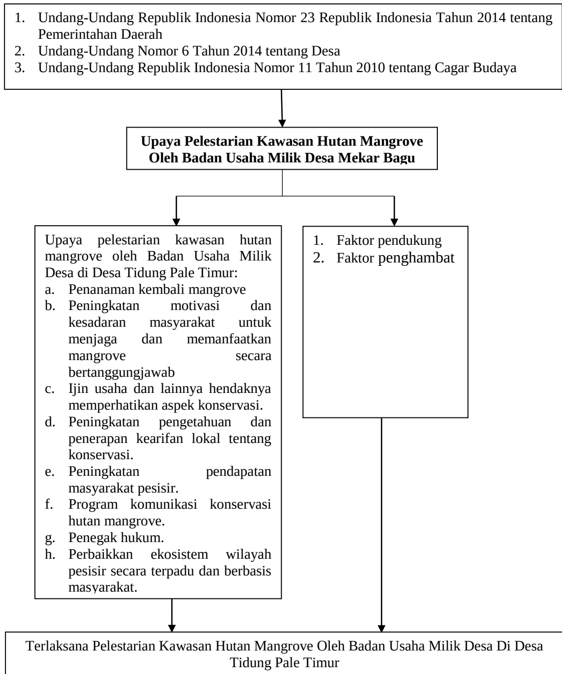
Gambar 2.1. Kerangka Pemikiran
